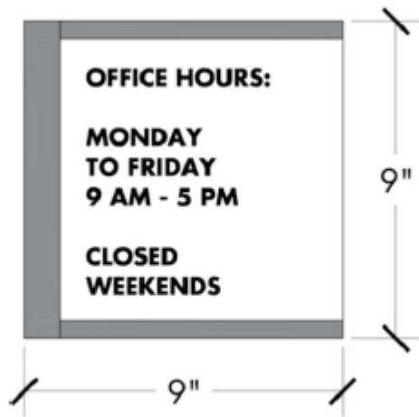
Scale: 3" = 1'-0"
